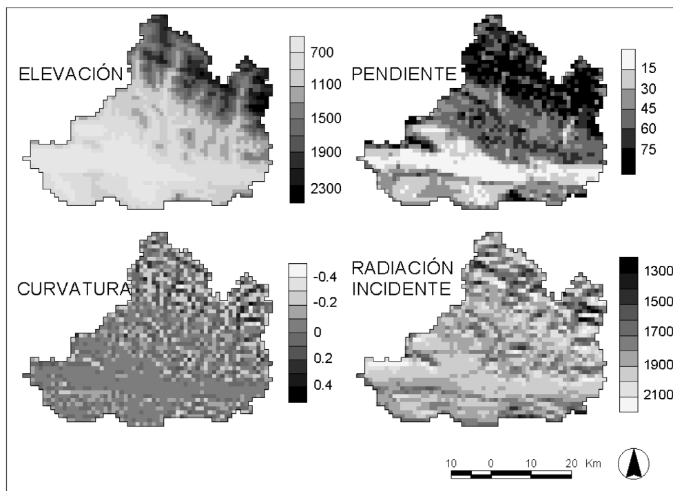
Figura 2. Factores topográficos. Elevación (datos en metros). Pendiente (datos en porcentajes). Curvatura ( \text{m}^{-1} ). Radiación solar incidente media anual ( \text{Kj m}^{-2} \text{sg}^{-1} \text{ día} ).
